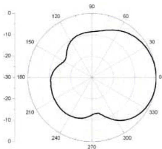
E Plane(90° )
