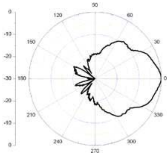
E Plane(40° )
