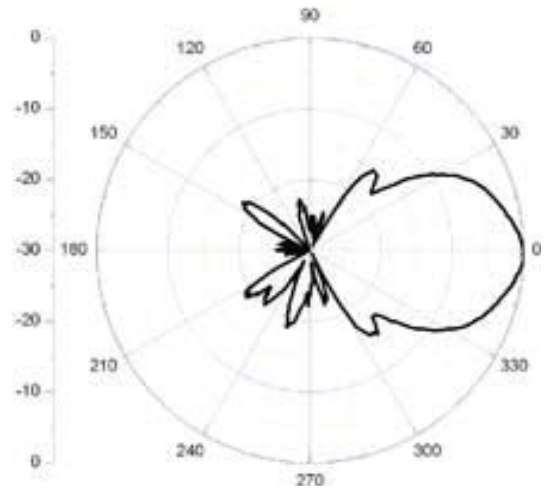
H Plane(34° )
