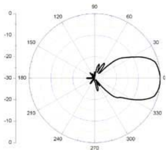
H Plane(34° )
