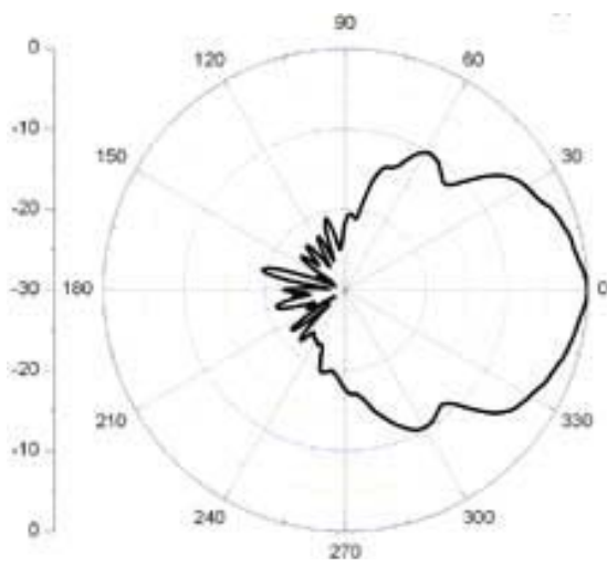
E Plane(40° )
